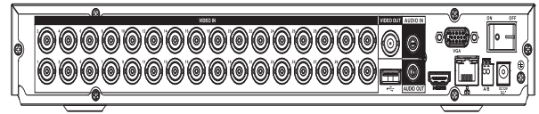
DHI-HCVR4232AN-S3
